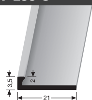
Abschlussprofil Edge trim
