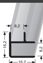
Clip-Außenecke Clip external corner
