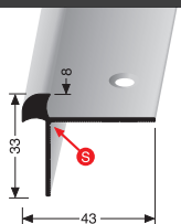
Treppenkantenprofil Stair nosing
