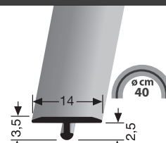
T-Profile T-profiles
