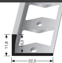
Doppel-K Profil Perforated edge trim
