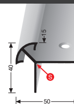
Treppenkantenprofil Stair nosing
