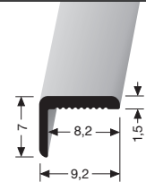
Winkelprofil Angle edge
