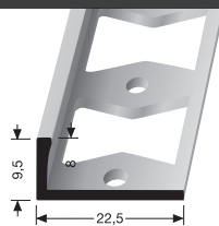
Doppel-K Profil Perforated edge trim
