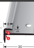
Treppenkantenprofil Stair nosing
