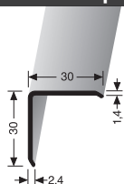
Eckschutzwinkel Corner guard
